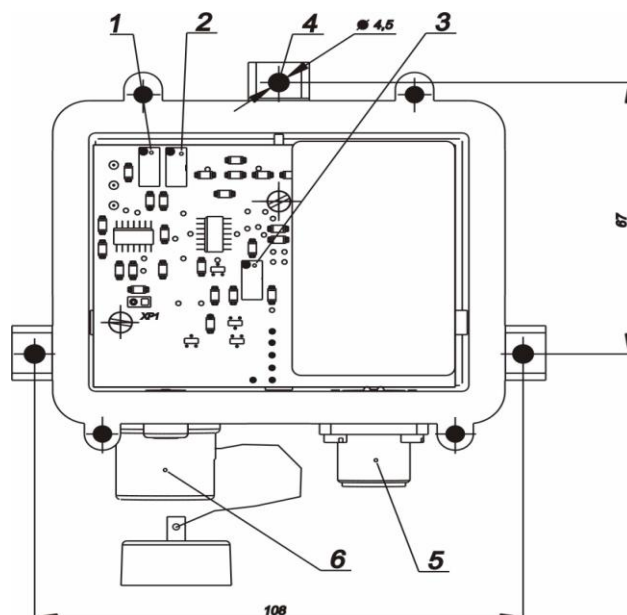
Рис.3.Датчик СИГМА-03.ДВ со снятой крышкой, присоединительные размеры. 1-потенциометр балансировки моста, 2-потенциометр регулировки начального тока, 3- потенциометр регулировки усиления, 4 – установочные отверстия диаметром 4.5 мм, 5 –розетка питания 6 – сенсор.
