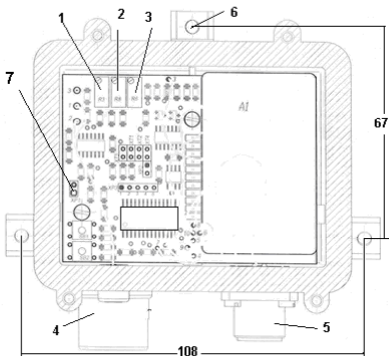
Рис.3. Датчик со снятой крышкой.
